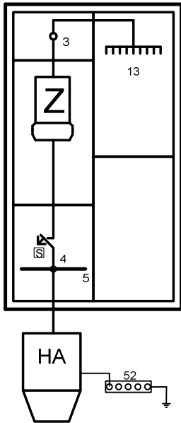
P 1.01 Einkundenanlage (z.B. Einfamilienhaus)
