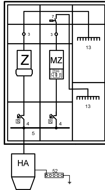
P 1.06 Einkundenanlage mit Freigabe- steuerung (Einfamilienhaus) TSG intern im Mehrtarifzähler
