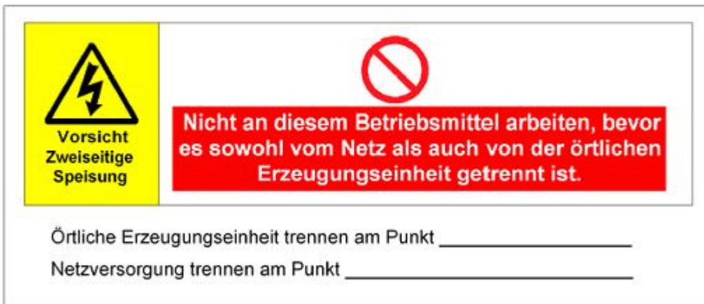
Abb. 6: Beispiel für einen Warnhinweis am Netzanschluss beim Anschluss einer Erzeugungsanlage gemäß DIN EN 50438
