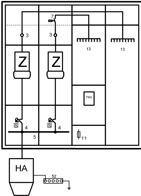
P 1.05 Einkundenanlage mit Freigabe- steuerung (Einfamilienhaus) TSG extern
