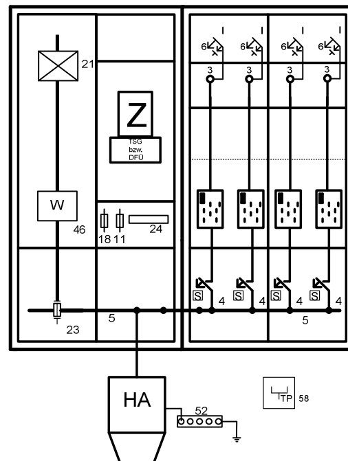
P 4.03 Mehrkundenanlage einstöckige Bauweise ohne Wechseltafel mit Zählerplatzflächen mit BKE-I (z.B. Wohn- und Geschäftshaus)
