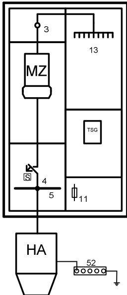
P 1.03 Mehrtarifzähler mit Tarifumschaltung (z.B. Einfamilienhaus)
