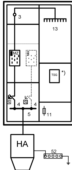
P 1.04 Mehrtarifzähler mit Tarifumschaltung (z.B. Einfamilienhaus)
