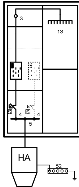
P 1.02 Einkundenanlage (z.B. Einfamilienhaus)
