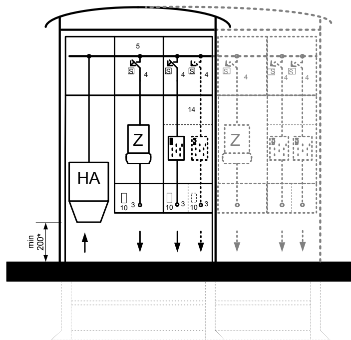
B 2.22 (Ausführung alternativ für eHZ oder Zähler mit Dreipunktbefestigung)
