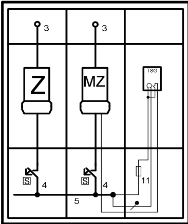
S 2.01 (Mehrtarifzähler mit externem TSG)
