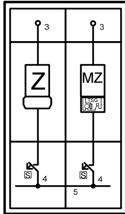
S 2.02 (Mehrtarifzähler mit internem TSG)
