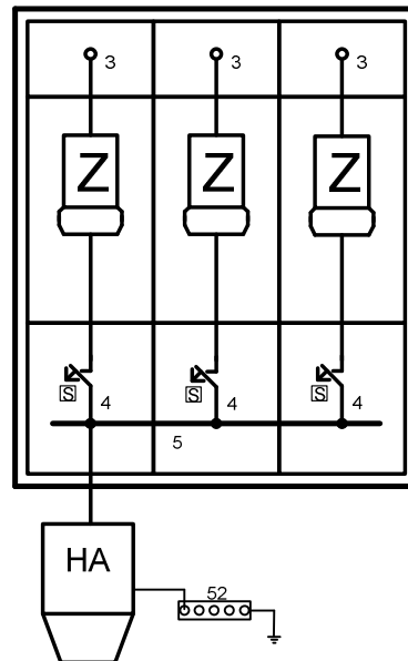
P 1.08 Mehrkundenanlage einstöckige Bauweise (z.B. Wohnhaus)
