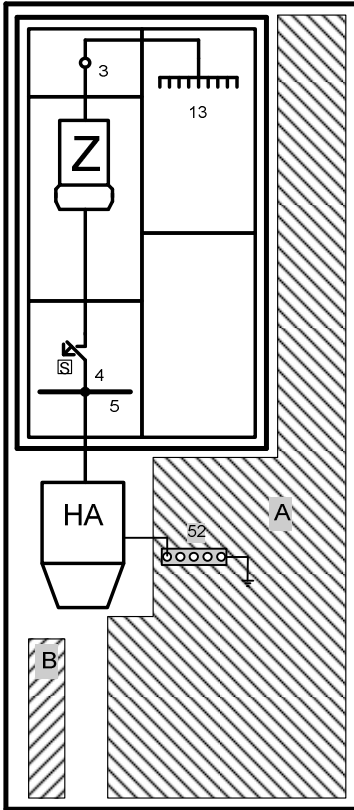
P 2.01 Einkundenanlage (z.B. Einfamilienhaus) für Zählerplatzflächen mit Drei-Punkt-Befestigung
