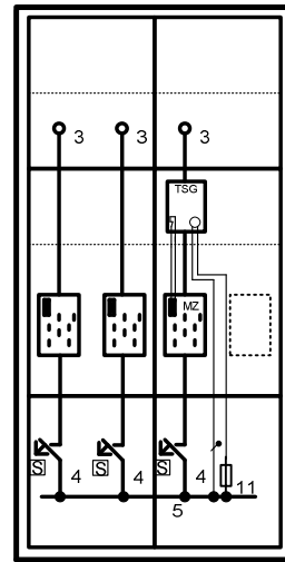
S 2.03 (Mehrtarifzähler mit TSG im Raum für Zusatzanwendungen)
